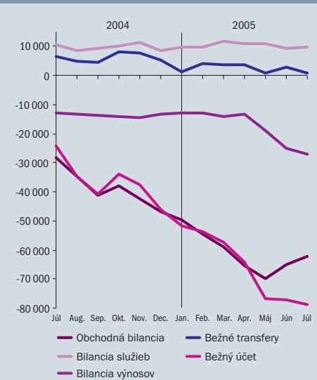
Graf 7 Vývoj bežného účtu a jeho zložiek (kĺzavé kumulatívy) (mil. Sk)
