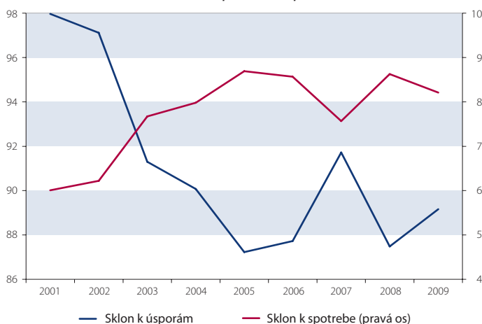
Graf 12 Sklon domácností k úsporám a spotrebe (v %)
