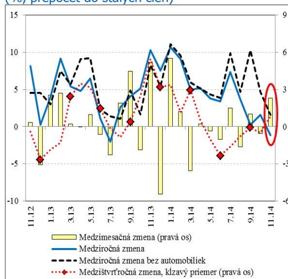
Export tovarov (%, prepočet do stálych cien)
