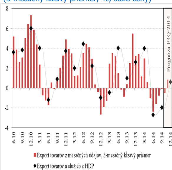
Medziročný vývoj exportu vybraných odvetví (3-mesačný klzavý priemer, %, stále ceny)
