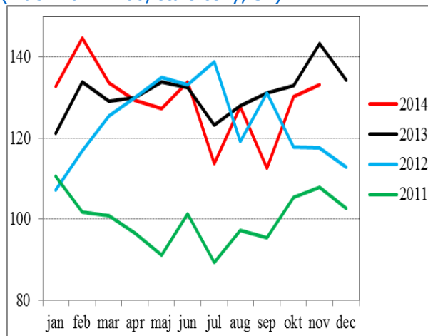
Export áut a príslušenstva (index 2011=100, stále ceny, SA)
