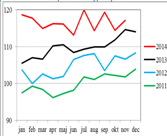
Export ostatných tovarov bez áut a príslušenstva (index 2011=100, stále ceny, SA)
