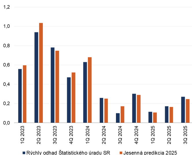
Graf 1 Vývoj reálneho HDP a predikcia NBS (medzištvrtročná zmena v %, s. o.)
