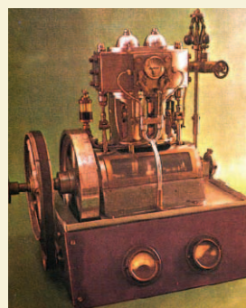
▲ Model parného dvojvalcového motora Model of a two-cylinder steam engine
