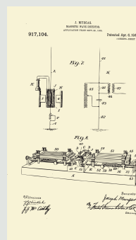
▲ Niektoré patenty Jozefa Murgaša Jozef Murgaš's patents
