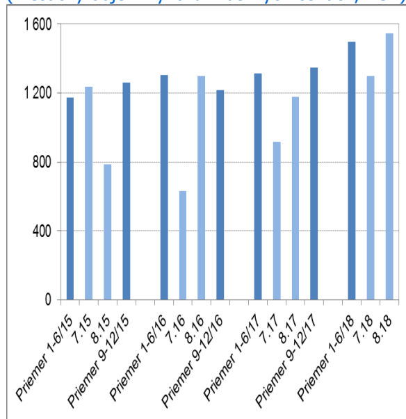
Graf 2. Letné dovolenky ovplyvňujú vývoz aut (mesačný objem vývozu v bežných cenách, NSA)
