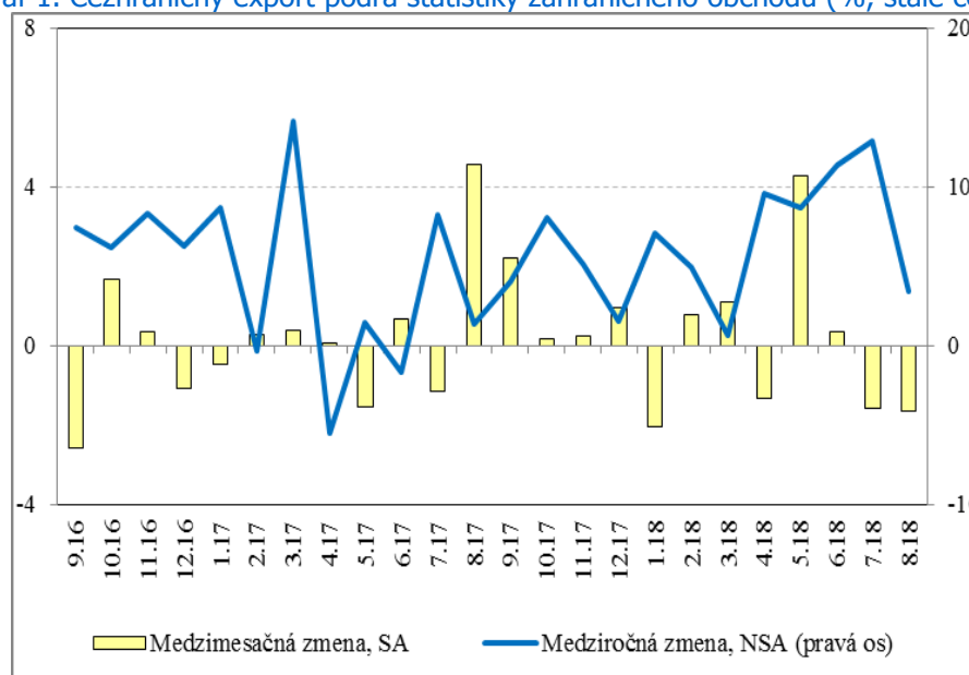
Graf 1. Cezhraničný export podľa štatistiky zahraničného obchodu (% , stále ceny)
