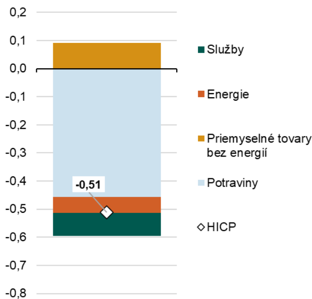
Graf 2 Štruktúra marcovej chyby jarnej predikcie (príspevky v p. b.)
