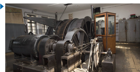
▶ Ťažný stroj na zvislú dopravu
